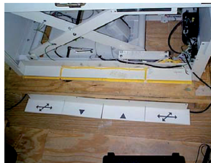
Nožní spínače u výškově nastavitelných stolů
